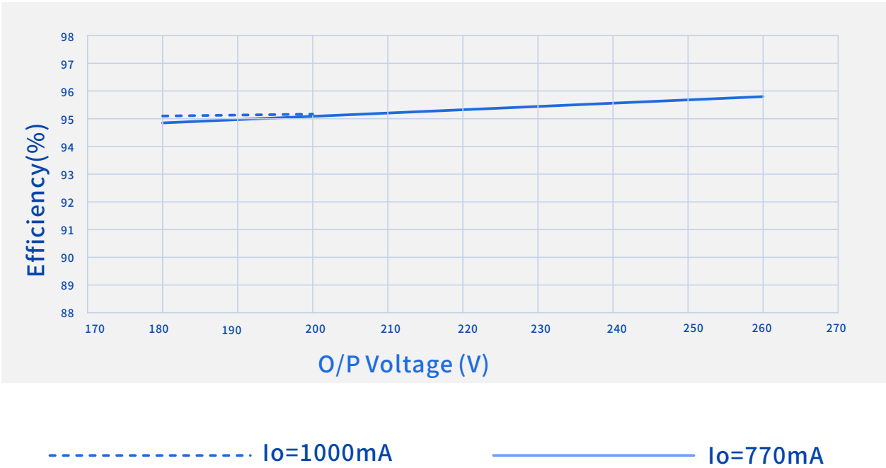
效率 Vs. 输出电压 (Vin=264Vac)
